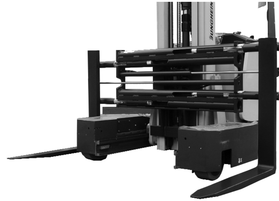
Integriertes Zinkenverstellgerät auf Klammerkörperbasis über den Fahrzeugrahmen hochgebaut
