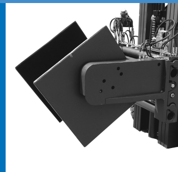
Paket-Kippgerät
