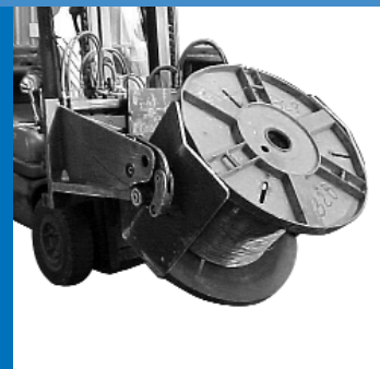
Kabeltrommel-Kippklammer – 180° kippbar
